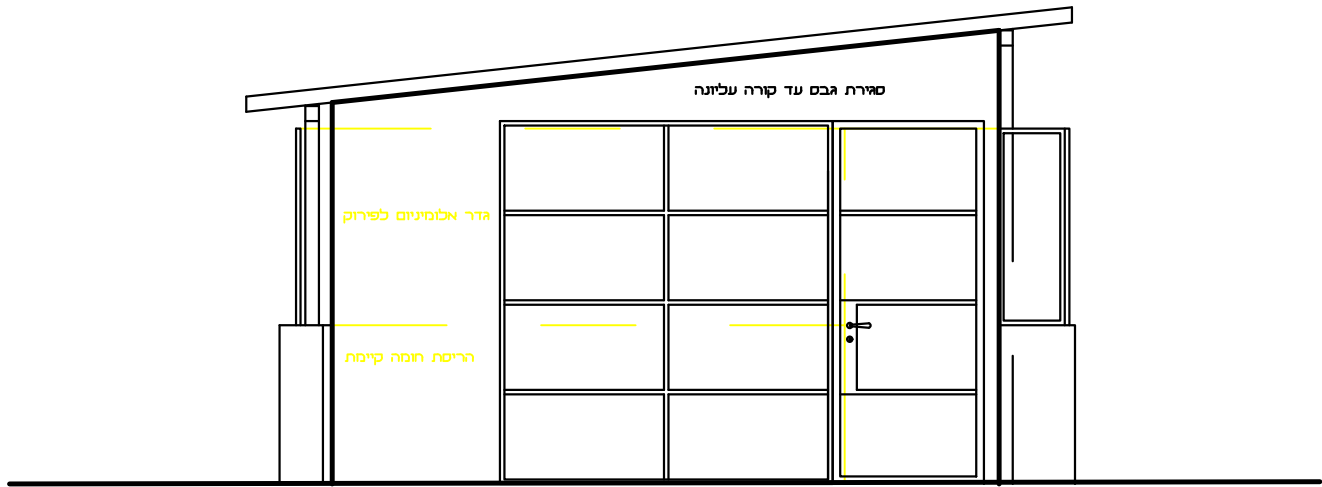
חזית כניסה קנ"מ 1:50
