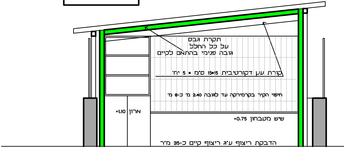
חזית קנ"מ 1:50
